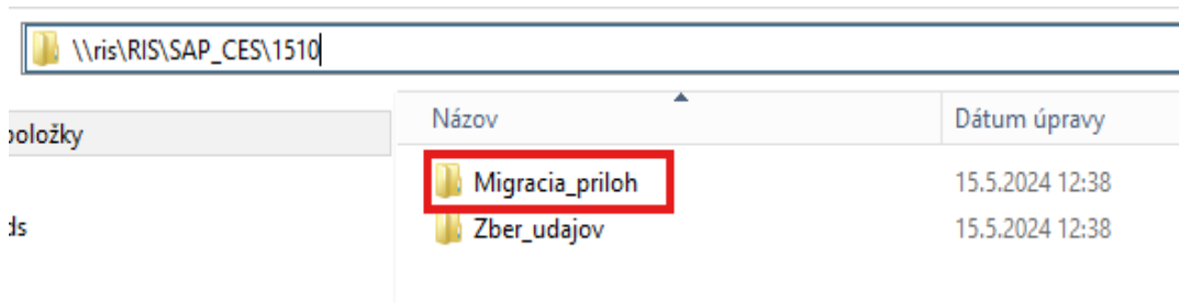
Obrázok 2 - Adresár
