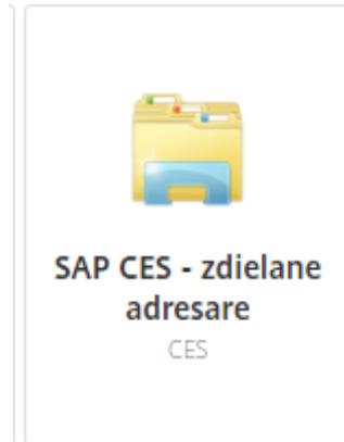
Obrázok 1 - Aplikácia
