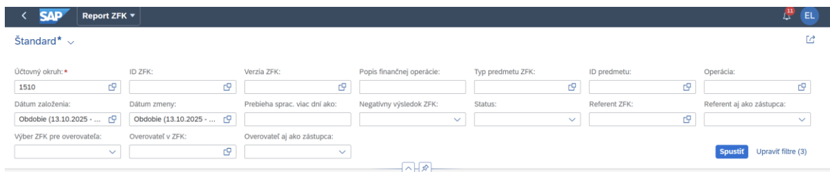
Obrázok 5 Vstupné parametre
