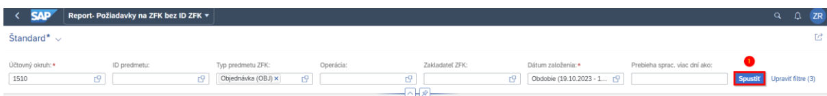
Obrázok 26 Spustenie reportu
