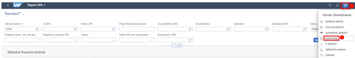
Obrázok 6 Fiori nastavenia
