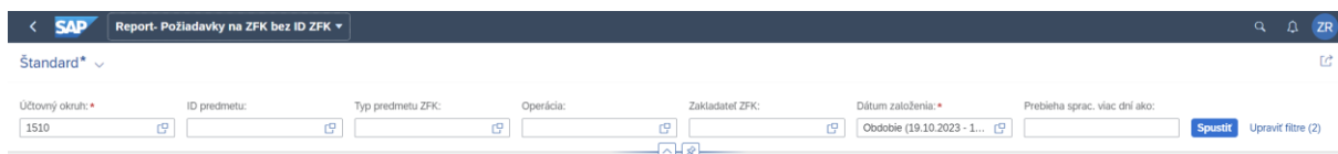
Obrázok 25 Vstupné parametre
