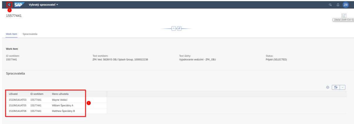
Obrázok 21 Spracovatelia Workflow
